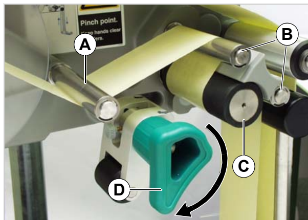
[41] Abrir el rodillo de presión.
