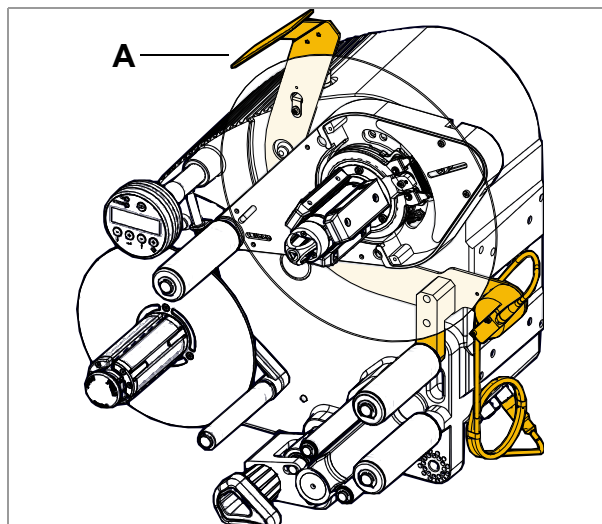
[17] Barrera óptica DR (A)
