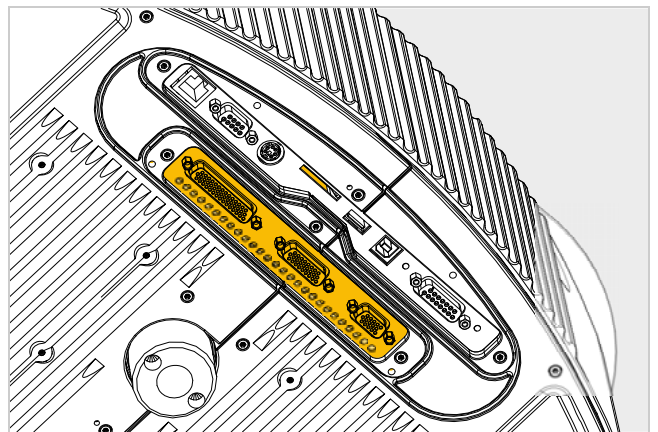
[21] Interfaz del aplicador.
