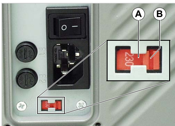
[30] Selector de tensión (ajuste en la ilustración: 230 V)
