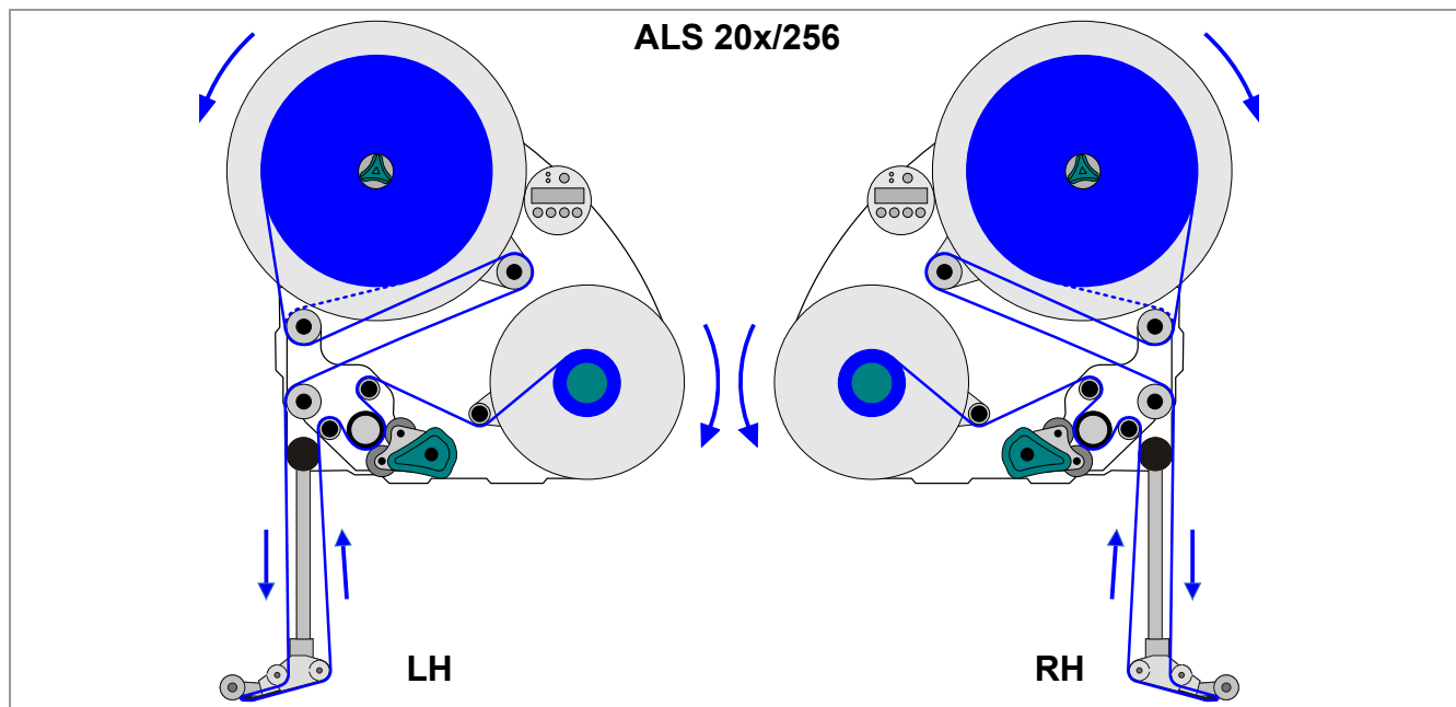
[35] Esquema de enhebrado para ALS 20x/256 con borde de dispensadora L
