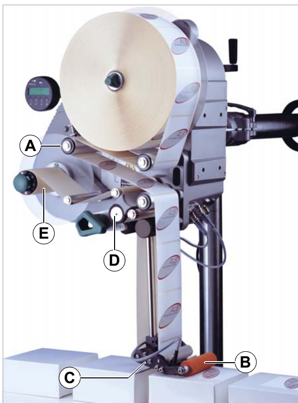
[4] Etiquetadora ALS 20x preparado para el servicio.
