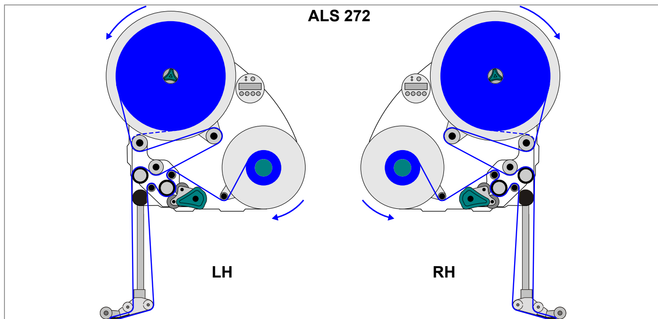
[36] Esquema de enhebrado para ALS 272 con borde de dispensadora L
