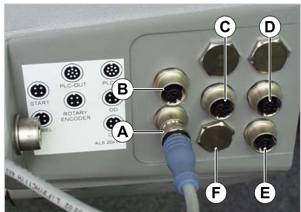
[32] Conexiones de los sensores:
