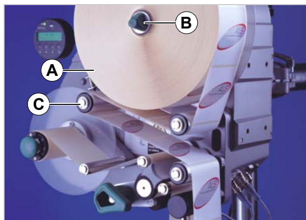
[34] Introducir rollos de material - Parte 1
